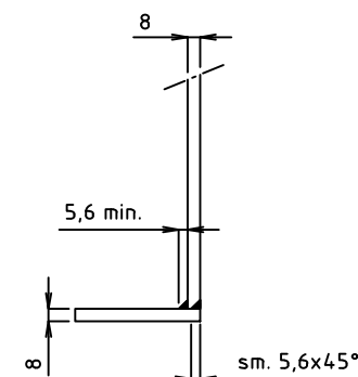
dettaglio saldatura piastra
