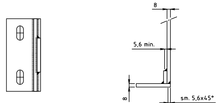
dettaglio saldatura piastra
