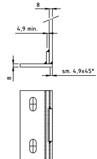
dettaglio saldatura piastra
