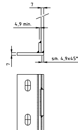
dettaglio saldatura piastra
