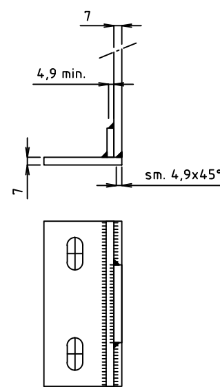
dettaglio saldatura piastra
