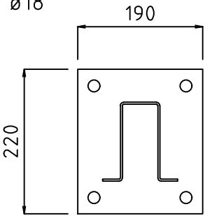
DIMENSIONE PIASTRA DI BASE FORI ø18
