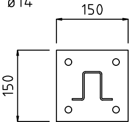
DIMENSIONE PIASTRA DI BASE FORI ø14
