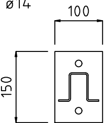
DIMENSIONE PIASTRA DI BASE FORI \varnothing 14
