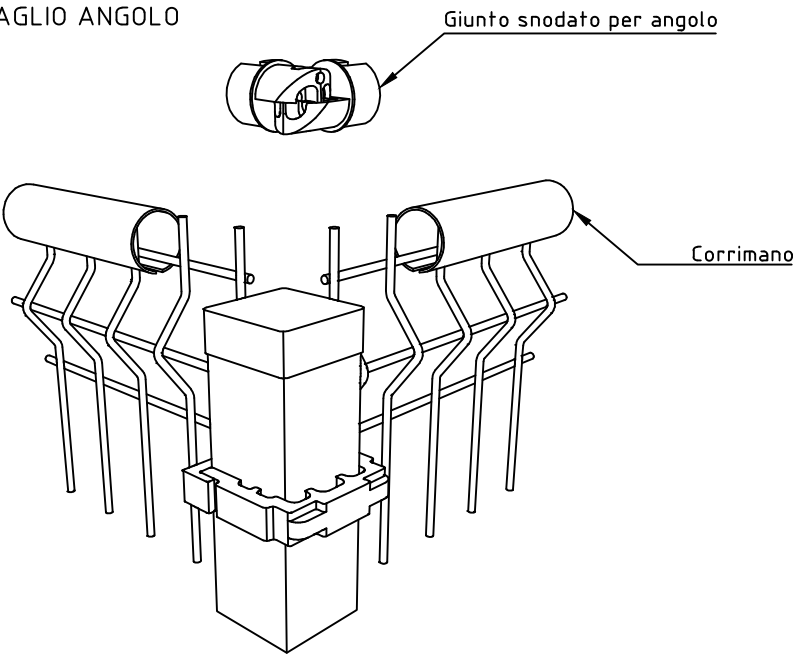
DETTAGLIO ANGOLO
