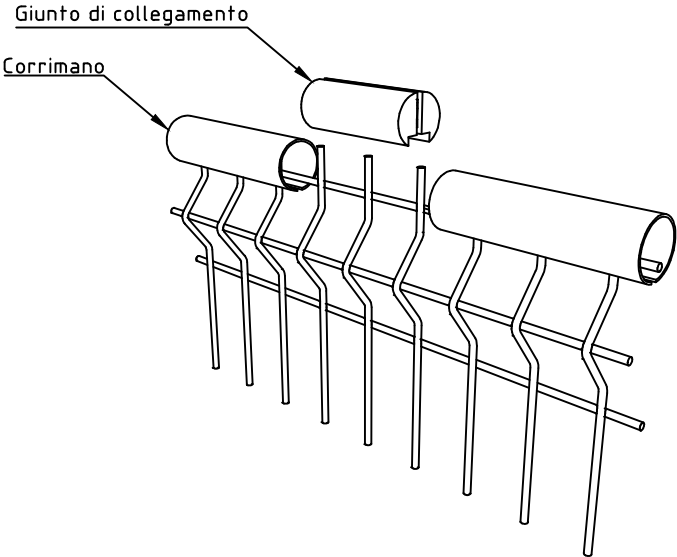
DETTAGLIO CORRIMANO
