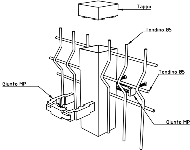
INSTALLAZIONE TIPO B PANNELLO IN LUCE
