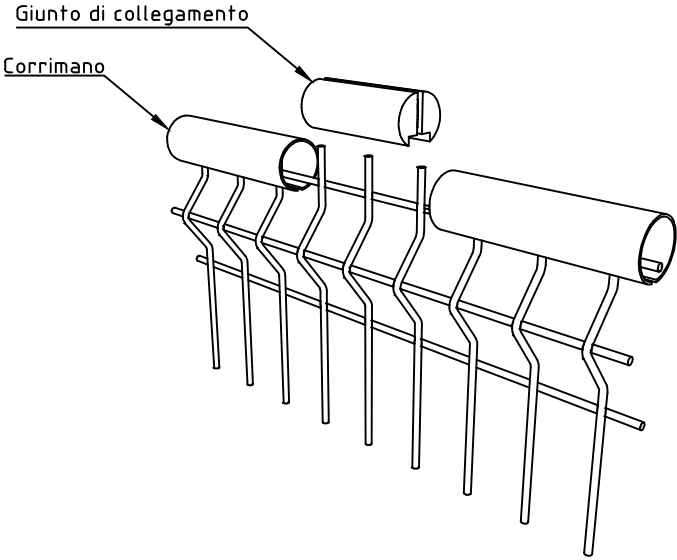
DETTAGLIO CORRIMANO
