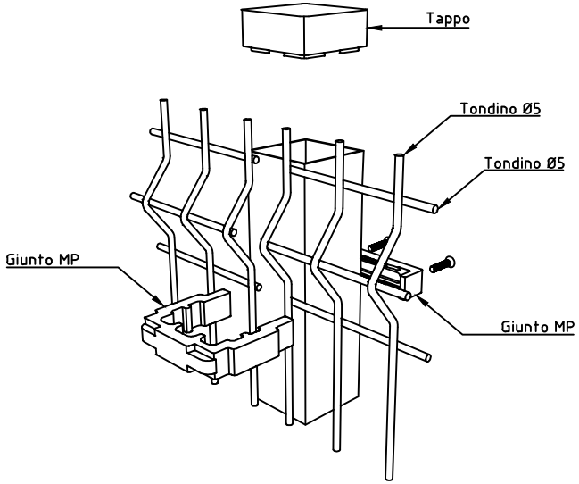
INSTALLAZIONE TIPO B PANNELLO IN LUCE
