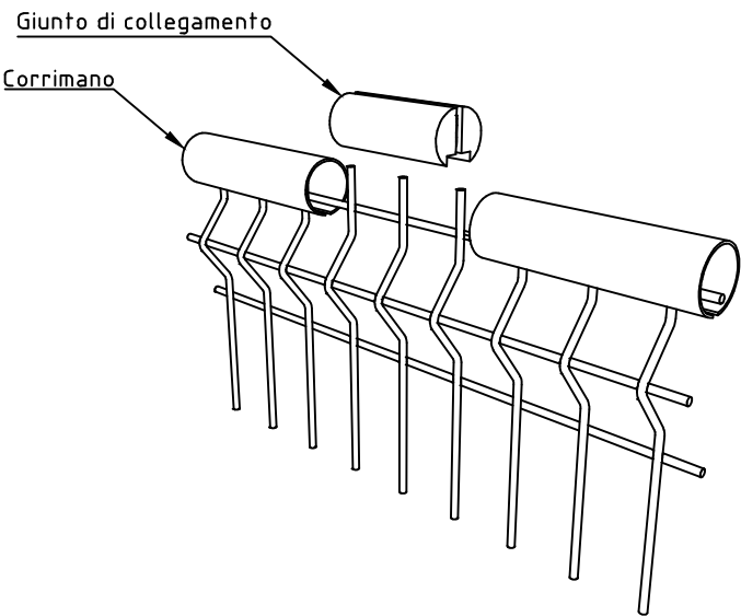
DETTAGLIO CORRIMANO
