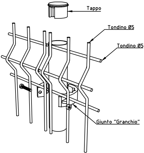
INSTALLAZIONE TIPO B PANNELLO IN LUCE
