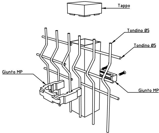
INSTALLAZIONE TIPO B PANNELLO IN LUCE
