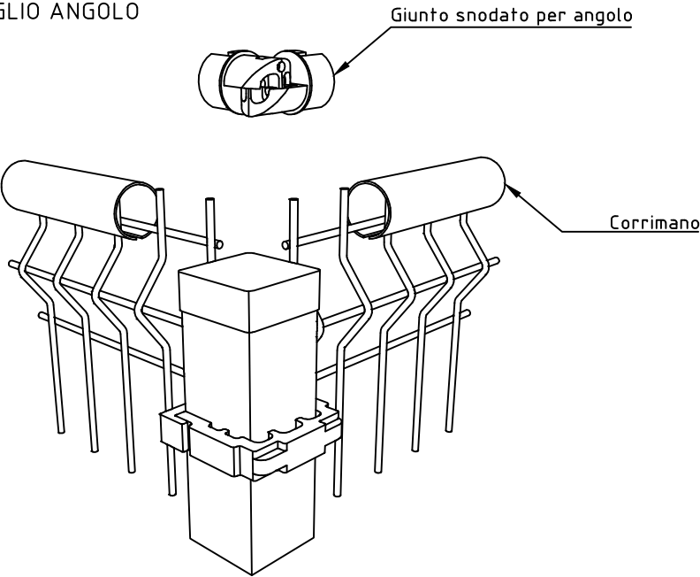
DETTAGLIO ANGOLO
