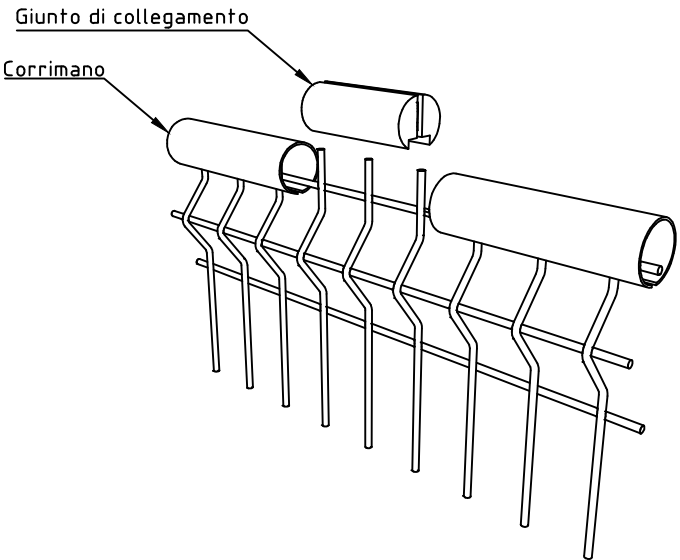
DETTAGLIO CORRIMANO
