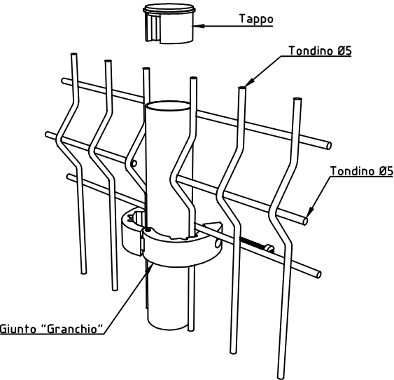
INSTALLAZIONE TIPO B PANNELLO IN LUCE
