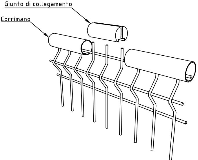
DETTAGLIO CORRIMANO
