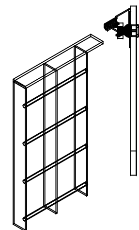
SQUADRETTA TELESCOPICA 45°
