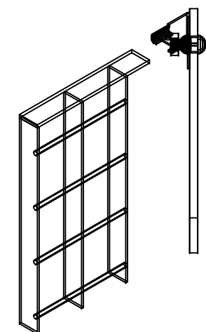
SQUADRETTA TELESCOPICA 45°
