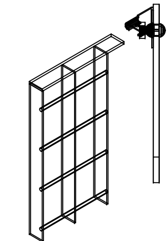
SQUADRETTA TELESOPICA 45°
