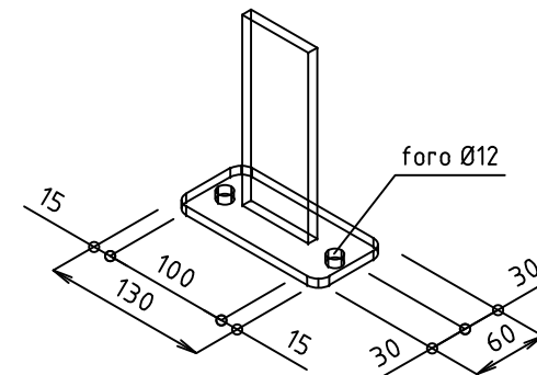
PIANTANA -60x7 lg. 1803 (da tassellare) kg/cad 7,1 DIMENSIONE PIASTRA 130x60x7
