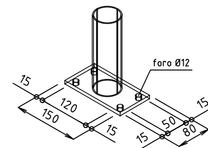
PIANTANA TUBO Ø60 SP.2 lg. 2100 (da tassellare) kg/cad zn. 6,0 DIMENSIONE PIASTRA 150x80x8
