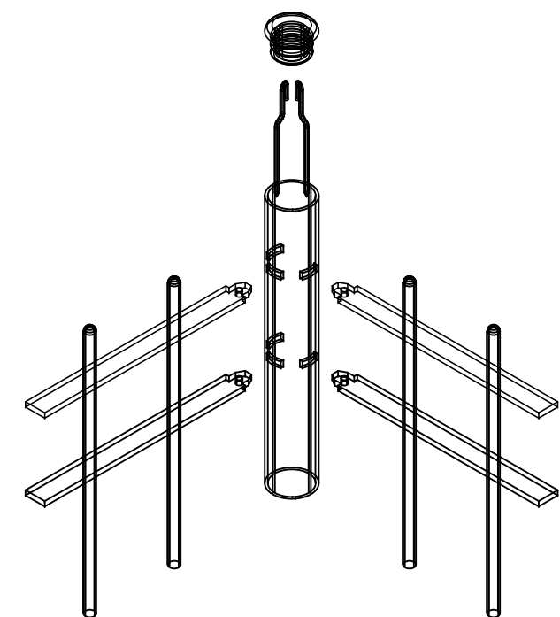
PART. ATTACCO ANGOLO 90°
