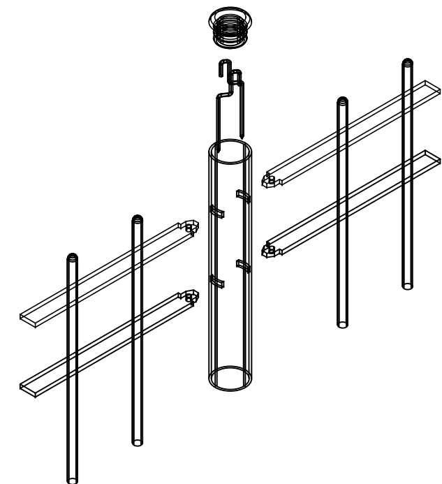
PART. ATTACCO INTERMEDIO
